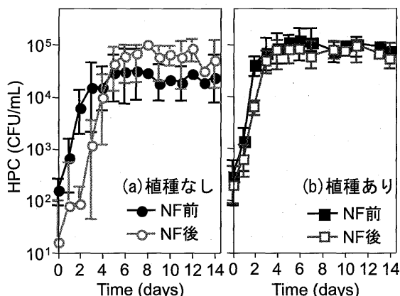
図4 膜処理前後の微生物学的安定性の比較 (a: 植種なし (n=8), b: 植種あり (n=6))
