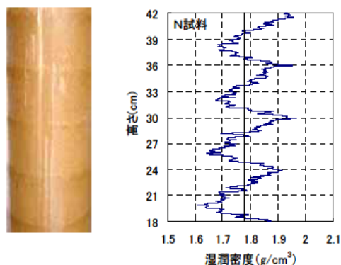
図 12 高松塚古墳の版築再現試験結果 7)
