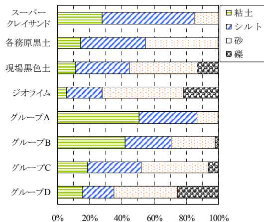
図 18 粒度組成（墳丘土，復元用土）
