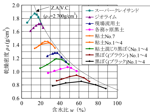
図 20 締固め試験結果 (填丘土、復元用土)
