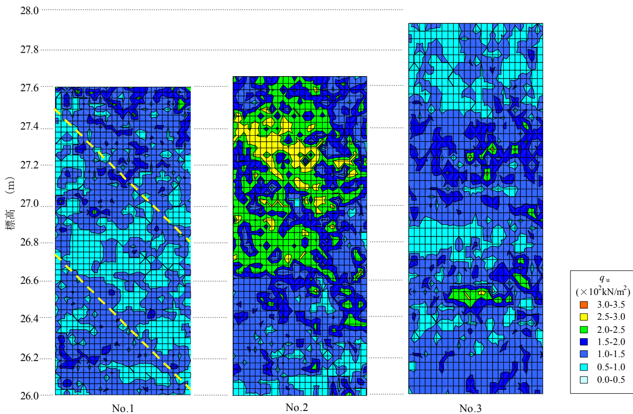
図 27 くびれ部の強度コンター図
