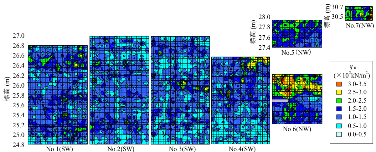
図 8 前方部南西側および北東側断面における換算一軸圧縮強さ分布
