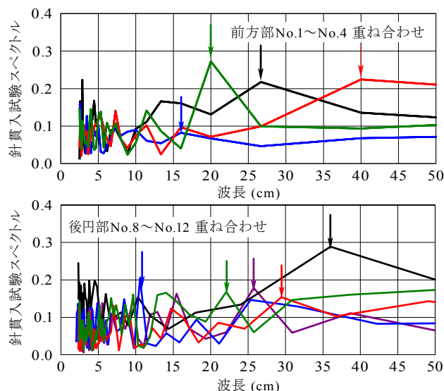
図 13 墳丘の強度変化の FFT 解析結果（上:前方部、下:後円部）
