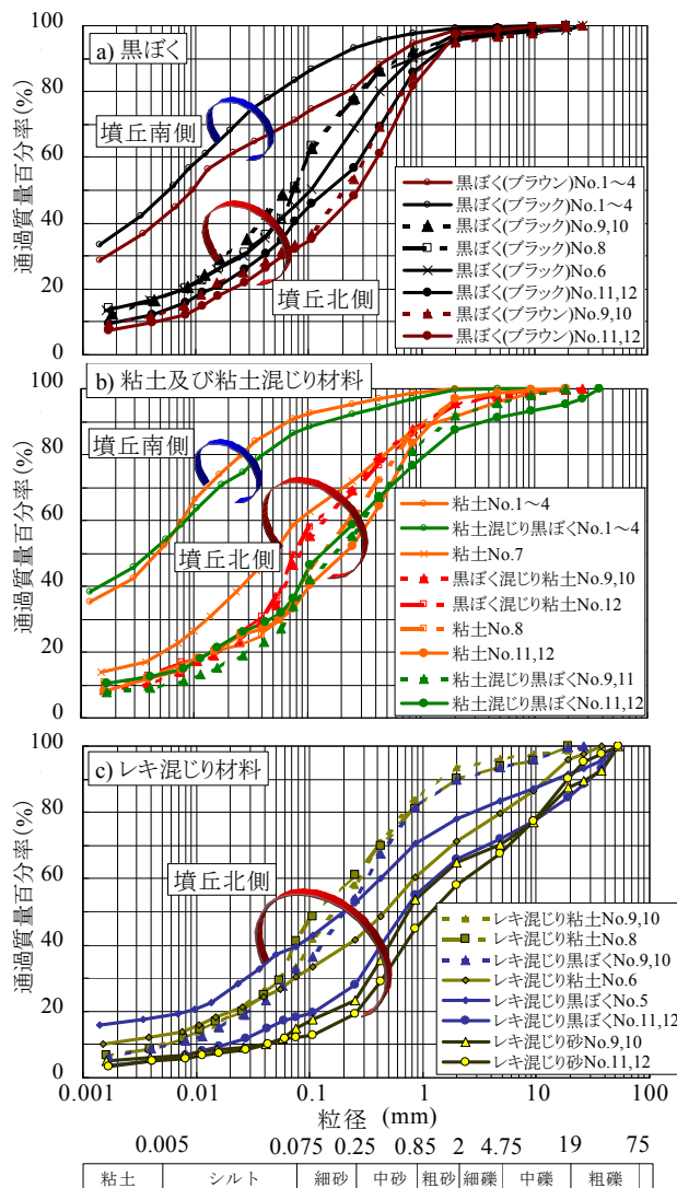
図 16 材料区分毎の粒度特性
