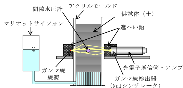
図 21 水分保持特性試験装置
