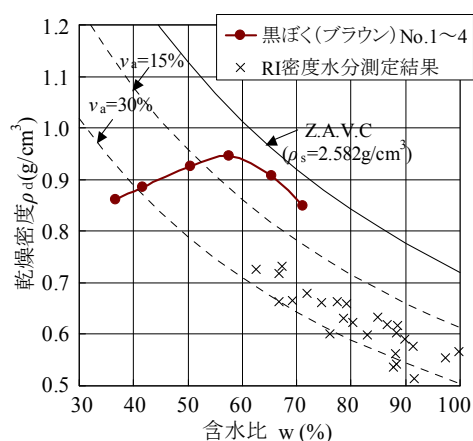
図 23 填丘土の締固め度（黒ぼく（ブラウン）前方部）
