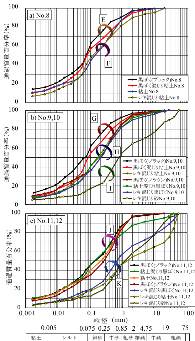
図 15 後円部を構成する材料の粒度特性
