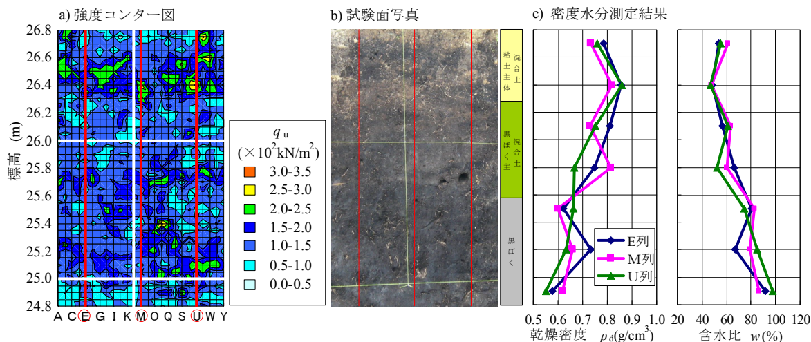
図 6 前方部試験エリア No.1 での調査試験結果
