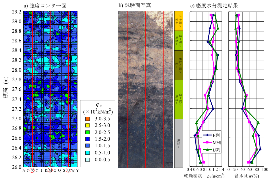
図 7 後円部試験エリア No.9 での調査試験結果
