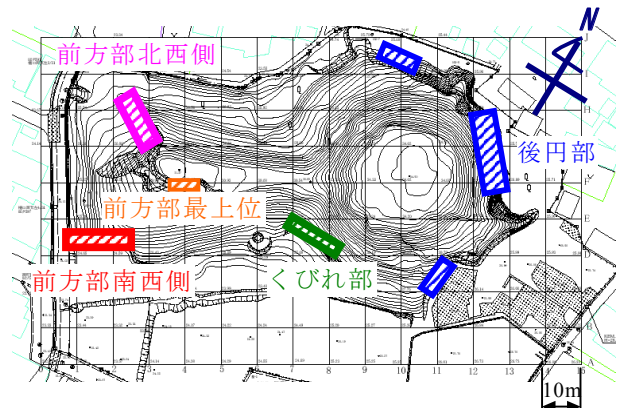
図 2 昼飯大塚古墳の地形と調査位置
