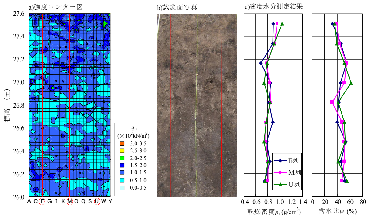
図 26 くびれ部試験エリア No.1での調査試験結果
