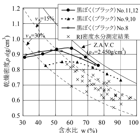
図 24 填丘土の締固め度（黒ぼく（ブラック）後円部）
