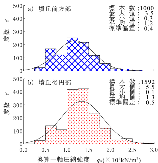
図 10 墳丘前方部と墳丘後円部の強度比較（黒ぼく）
