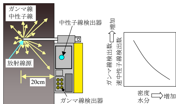
図 4 表面透過型 RI 密度水分計の概要
