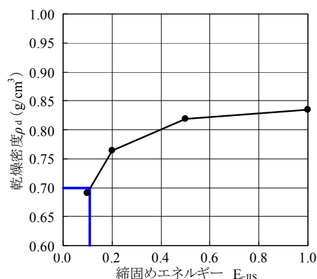
図 25 締固めエネルギーを変えた締固め試験結果
