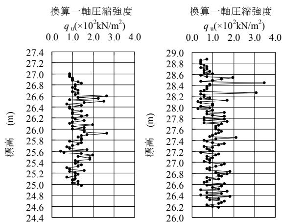
図 11 鉛直方向の一軸圧縮強度の変動（前方部 No.1、後円部 No.12）
