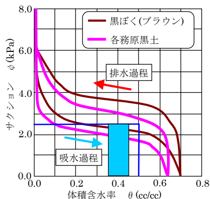
図22 水分保持特性試験結果
