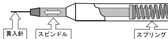
図 3 針貫入試験機
