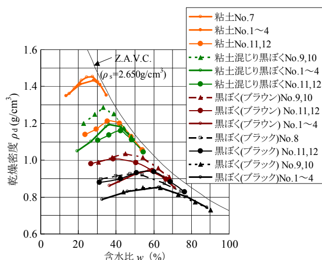
図19 締固め試験結果 (填丘土)
