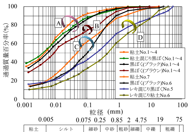
図 14 前方部を構成する材料の粒度特性
