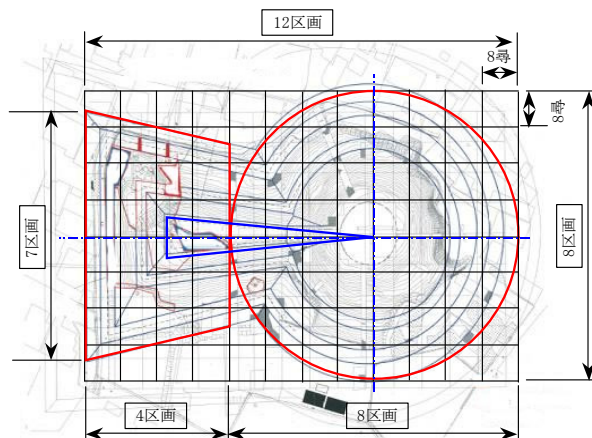
図 28 昼飯大塚古墳の設計
