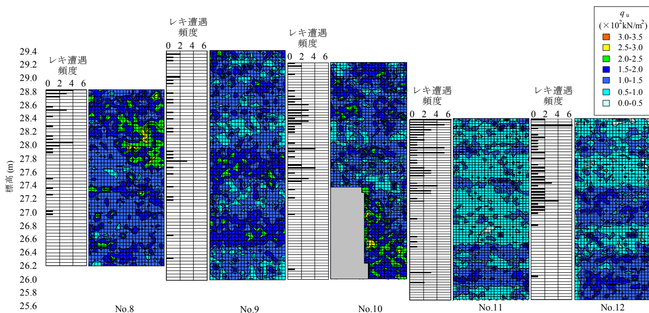
図 9 後円部の強度分布
