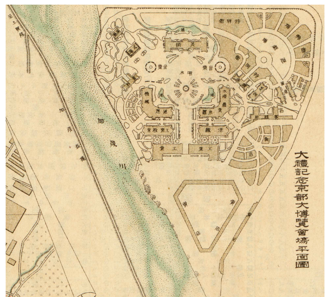
図4 「京都市街全圖」の線路図(上図: 原図記載の市營電鐵線路を赤線, 京都電鐵経路を黒線, 其他電鐵経路を青線で強調し文字を加筆, 下図: 博覽會平面図を拡大)
