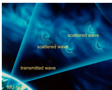
大気乱流からの散乱 対流圏/成層圏/中間圏
