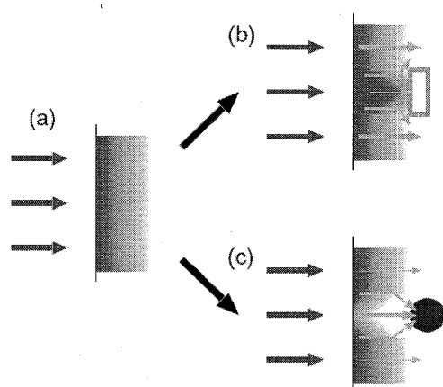
図1 加熱コンクリート中の熱伝導
