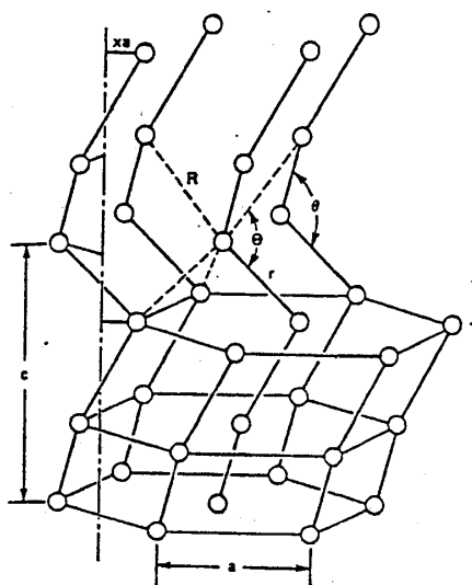
図〔4.8〕 trigonal Se
