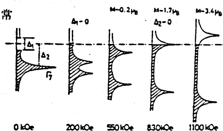
図-9 \text{YbB}_{12} のバンド構造模型
