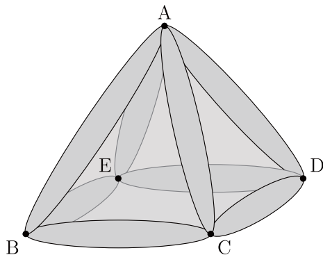
図 1 Hirzebruch 曲面上の複素直線束の Thom 空間
