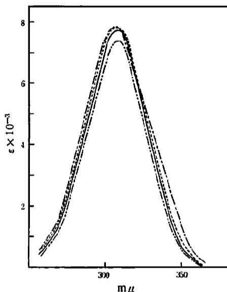
Fig. 7 Ultraviolet spectra of neopentoylformoin in tetrahydrofuran (—), acetonitrile (---), ethanol (····) and ether (— · — · —)
