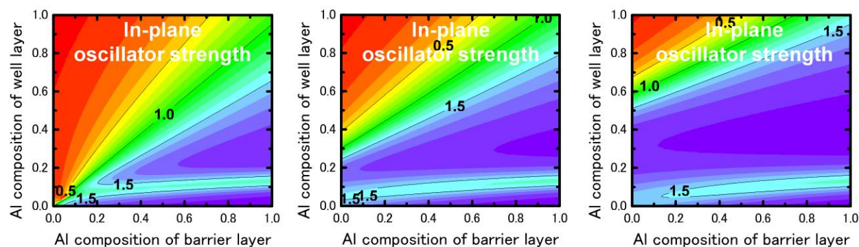
図 7.4 r 面 AlGa 0.5 N 0.5 /AlGa 0.5 N 0.5 歪み量子井戸構造の面内相対振動子強度の井戸幅依存性。
