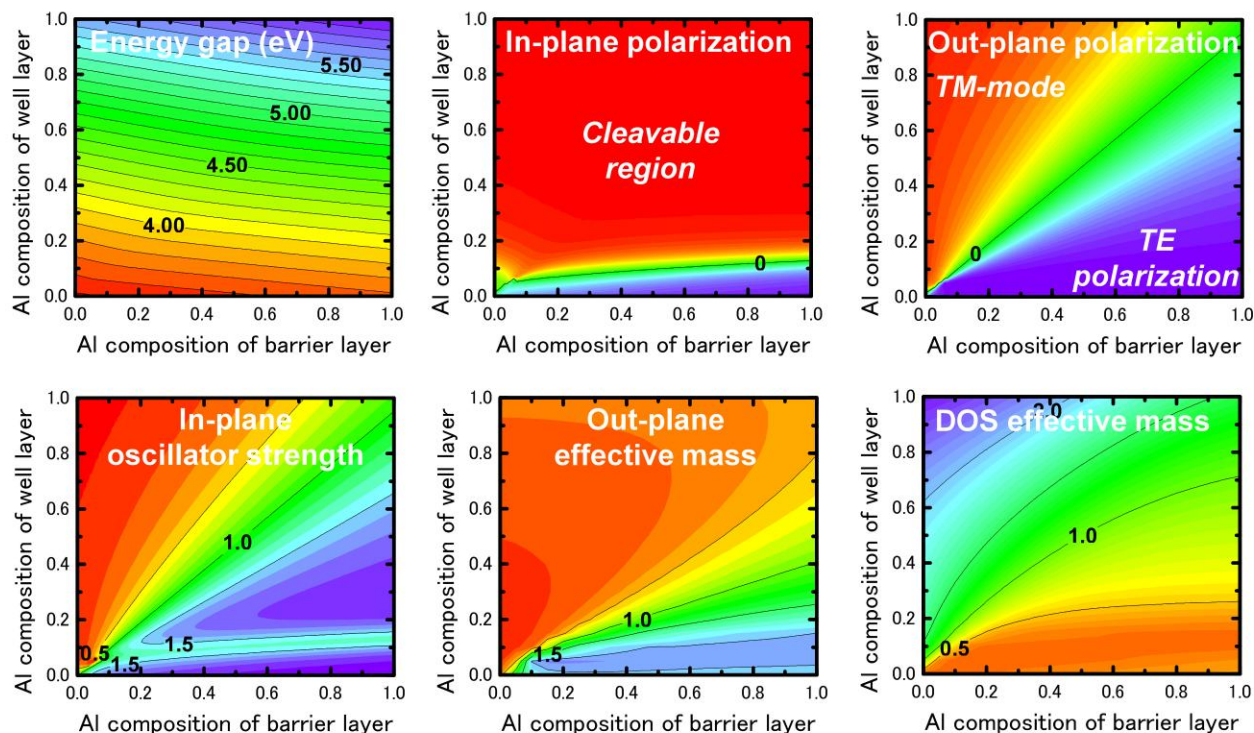
図 7.3 r 面 AlGa 0.5 N 0.5 /AlGa 0.5 N 0.5 歪みダブルヘテロ構造の禁制帯幅，面内偏光度と面外偏光度，面内相対振動子強度，面外有効質量と面内状態密度有効質量。
