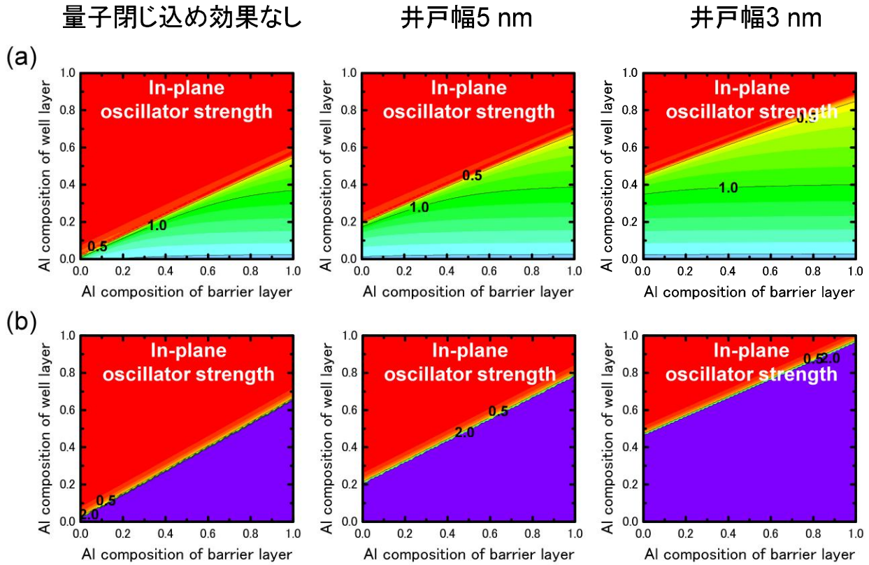
図 7.2 c 面 AlGaIn/AlGaIn 歪み量子井戸構造の面内相対振動子強度の井戸幅依存性. 赤色の部分の面内相対振動子強度の値は 0 である. (a) 本研究で同定した物性定数を用いて計算, (b) 参考文献 [35] の物性定数を用いて計算.
