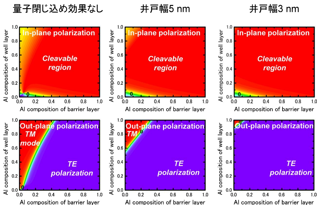
図 6.12 無極性面 AlGa N /AlGa N 歪み量子井戸構造における A 励起子遷移の偏光度の井戸幅依存性.
