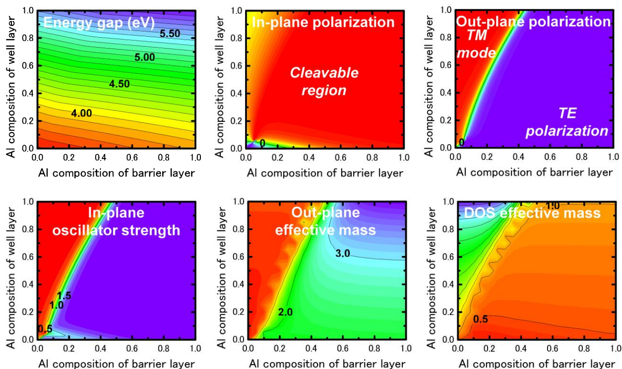
図 7.7 無極性面 AlGaIn/AlGaIn 歪みダブルヘテロ構造の禁制帯幅，面内偏光度と面外偏光度，面内相対振動子強度，面外有効質量と面内状態密度有効質量。
