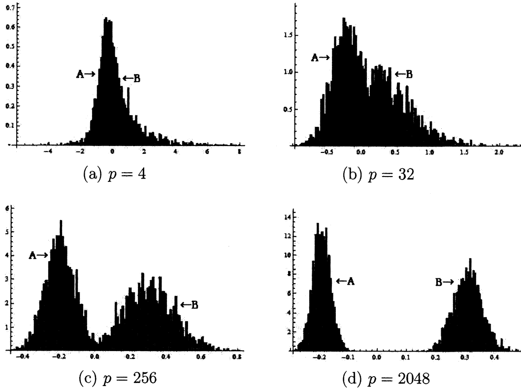
図1. \pi_1 : N_p(0, I_p) , \pi_2 : N_p(0, 2I_p) のとき, A : x_0 \in \pi_1 と B : x_0 \in \pi_2 に対する \omega(x_0) のヒストグラム.
