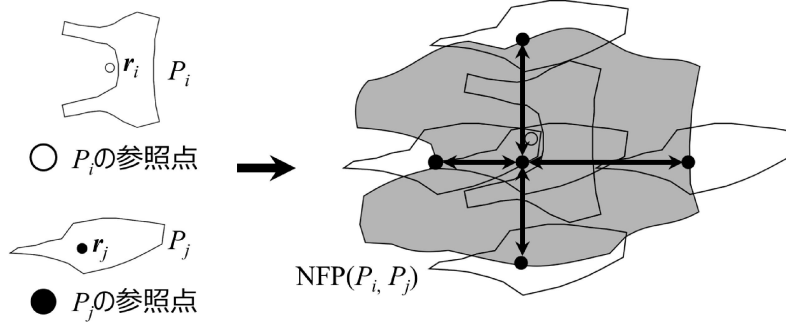
図 6: 図形 P_i, P_j に対するミンコフスキー差
