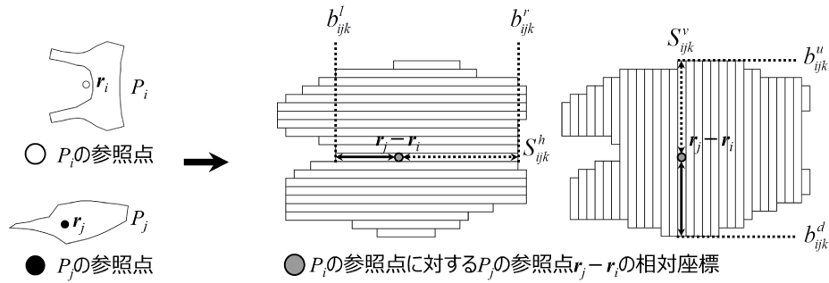
図 7: ミンコフスキー差による図形 P_i, P_j の重なり度 f_{ij}(r_i, r_j, o_i, o_j) の計算
