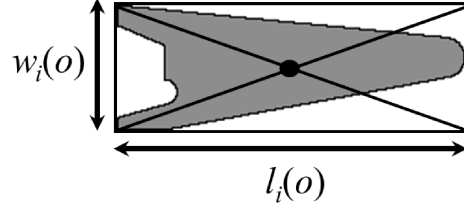
図 4: Bounding Box による参照点の決定
