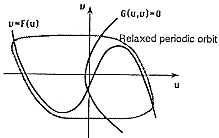
Figure 3: 周期解の存在
