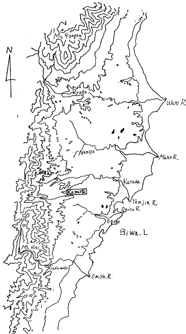
Fig. 1 Index map
