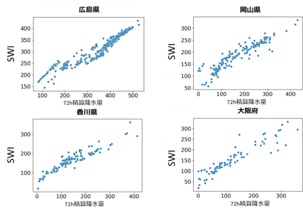
図 6 4 府県と 72h 積算降水量と SWI の関係 縦軸:72h 積算降水量 横軸:SWI
