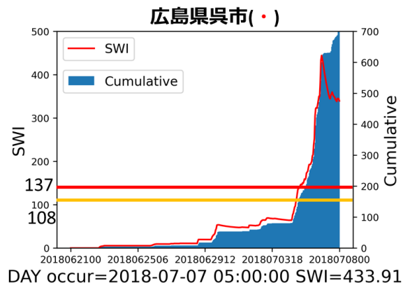
図2 西日本豪雨時の広島県呉市の土砂災害状況 下記の時間は土砂災害が起こった時刻 青棒グラフ:期間内の積算降水量 赤折れ線:SWI 変化 赤線:呉市の警報基準値 黄線:呉市の注意報基準値
