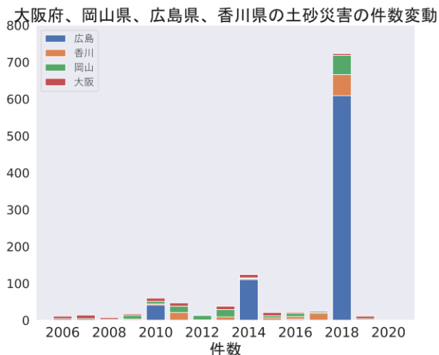
図1 4府県の土砂災害の件数変動 青色:広島 橙色:香川 緑色:岡山 赤色:大阪
