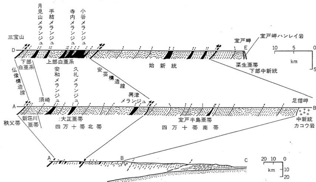
第7図 四国における四万十超層群の地質断面図〔メランジュ（黒色部）がサンドウィッチ状に粗粒碎屑岩相からなるスラスト・シートの上に挟まれる〕 （平，1990）
