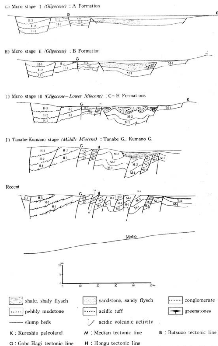
第 2 図 紀伊半島における四万十地尙斜の発展を示す模式図 (紀州四万十団体研究グループ, 1975) (K は黒潮古陸)
