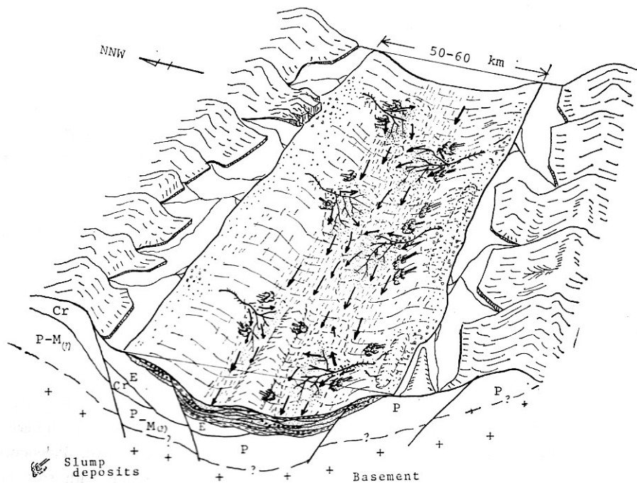
第3図 四万十超層群を形成した四万十地帯斜の復元の例 (Tateishi, 1978)
