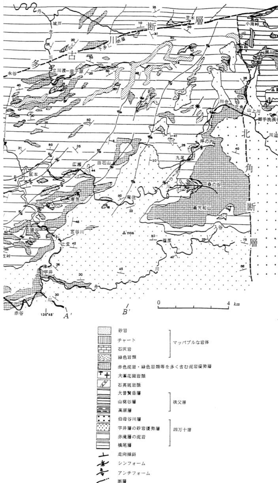
第12図 奈良県吉野郡辻堂地域の地質図 (大和大峰研究グループ, 1998 より) (槇尾層および赤滝層は日高川層群花園層に対比されるメラング相の付加体； 宇井層は日高川層群美山層に対比される粗粒碎屑岩相の付加体；南北性断層の 東側に粗粒碎屑岩相の付加体である湯川層に対比される伯母谷川層が分布する)
