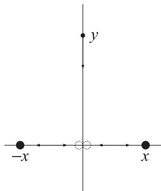
図 7 平面 Sitnikov 問題
