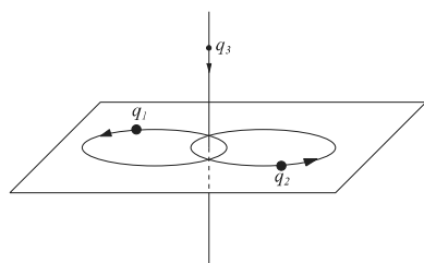
図 6 Sitnikov 問題
