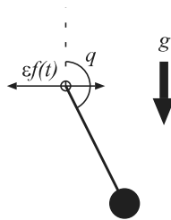
図 1 支点が周期運動する振り子
