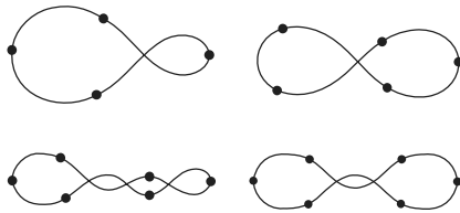
図4 鎖型舞蹈解
