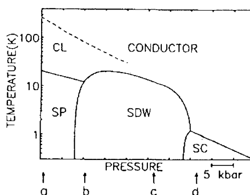
図 4 TMTSF 系における温度—圧力相図（文献 2）。SC:超伝導、SDW:スピン密度波、SP:スピンパイエルス相、CL:電荷局在（常磁性絶縁相）
