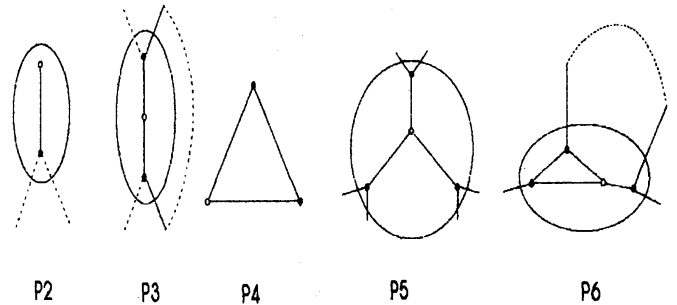
図 1: G(\mathcal{F}_\sigma) の分割
