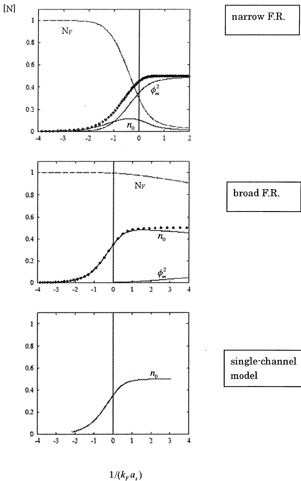
図 8. 4 : 凝縮粒子数 (点は全凝縮分子数=クーパー対+フェッシュバッハ分子)。 N_F は open channel の原子数。
