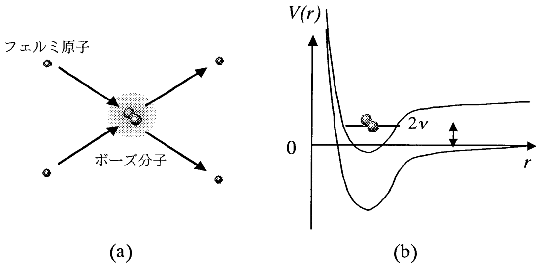
図4.3 : (a) フェッシュバッハ共鳴によって生じる引力相互作用 (b) 共鳴束縛状態形成の模式図
