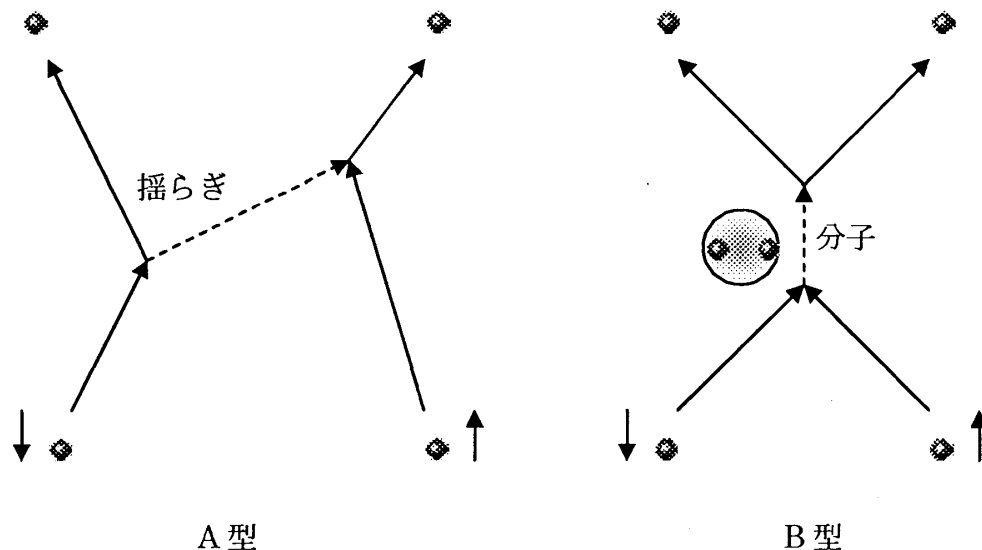
図4. 1： ボソンによって媒介（伝達）されるフェルミ粒子間相互作用
