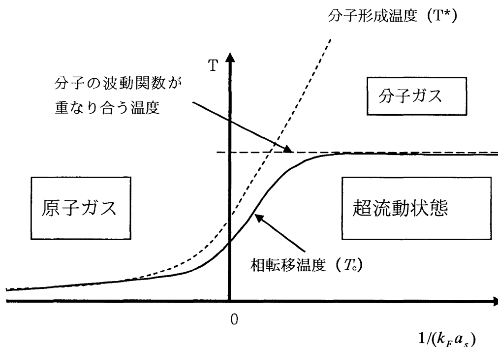
図 3. 7 : BCS-BEC クロスオーバーの相図
