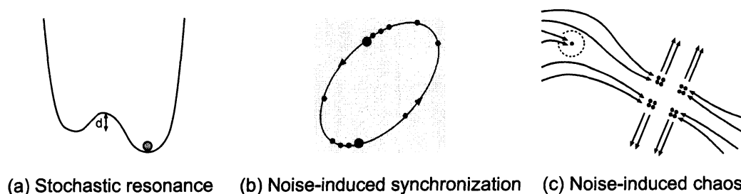
図 1: 雑音誘起現象の生じる力学系の状態空間の構造。(a) 確率共鳴: 勾配系のポテンシャルバリア。(b) ノイズ同期: 振動子系のリミットサイクル上の淀み構造。(c) 雑音誘起カオス: カオス的力学系のカオティックサドルと安定周期解。
