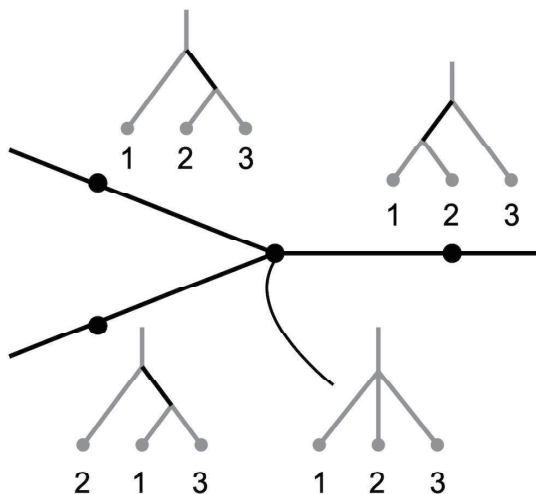
図1 3種の系統樹空間 (3-spider)
