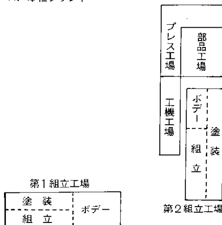
第2図 トヨタ車体工場配置 (1965年)
