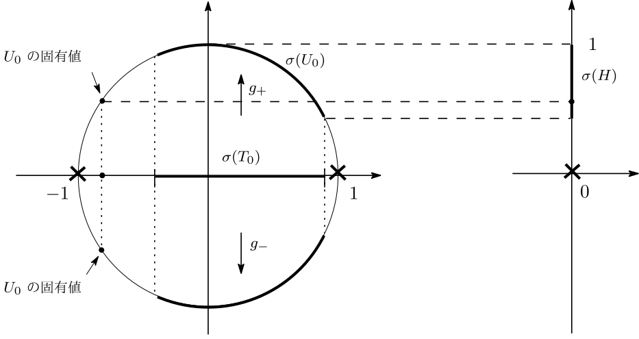
図3 U と H のスペクトルの関係.
