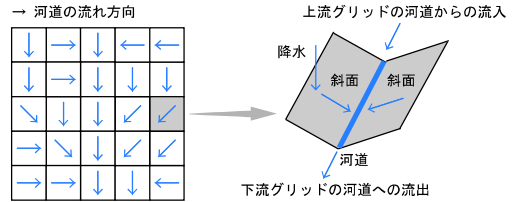
(a) 標高データを用いた河川の流下方向の設定(左)と一つの地形グリッド内での斜面と河川の地形モデル(右)
