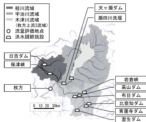
図-6 枚方地点上流域の流域モデル
