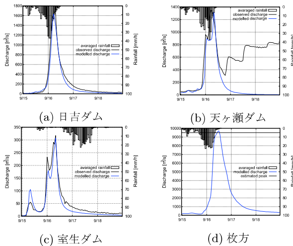
図-7 各地点での観測流量(枚方地点は推定ピーク流量)と再現計算流量
