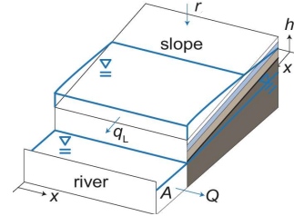
(b) 地形グリッド内での斜面流モデルと河川流モデル
