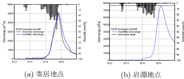
図-3 寄居地点の観測流量と再現計算流量, 岩淵地点の推定ピーク流量と再現計算流量
