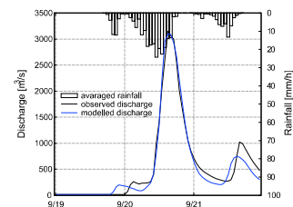
図-5 枇杷島地点の観測流量と再現計算流量
