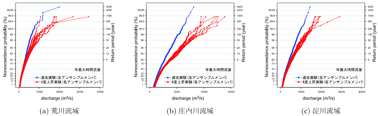
図-10 年最大時間流量の確率プロット (青線: 過去実験, 赤線: 4 度上昇実験 (SST 設定ごとに確率プロットを示す))
