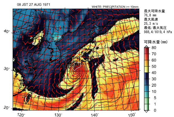
(b) 可降水量と海面気圧, 地上風速
