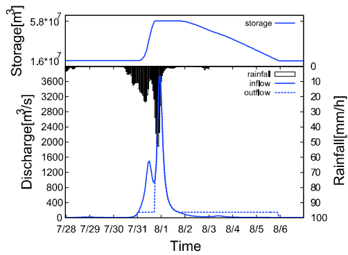
図-12 日吉ダムの流入量と放流量(下)と貯水量(上)
