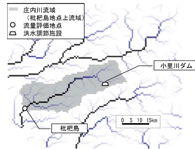
図-4 枇杷島地点上流域の流域モデル
