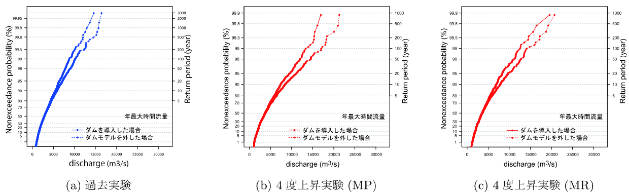
図-11 淀川流域枚方地点におけるダム貯水池の有無による年最大ピーク流量の確率プロットの比較
