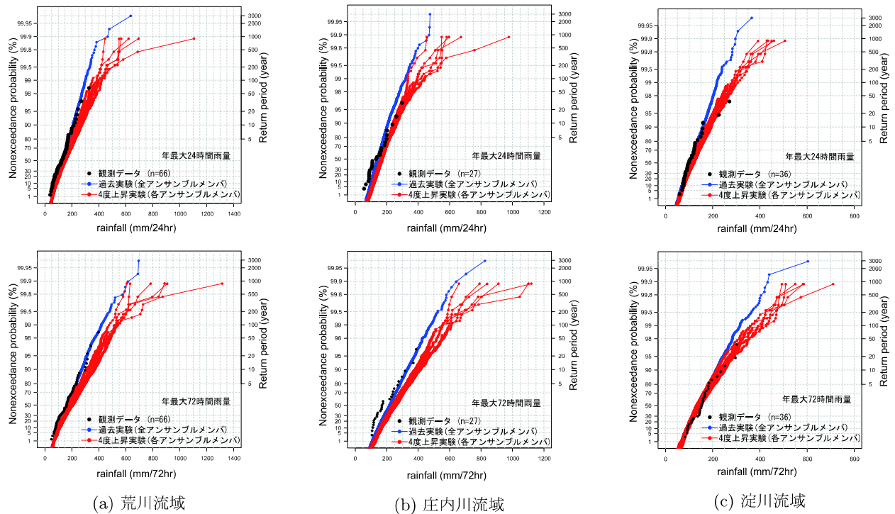
図-9 各流域の年最大24時間降水量(上段)と年最大72時間降水量(下段)の確率プロット(黒点:観測降雨,青線:過去実験,赤線:4度上昇実験(SST設定ごとに確率プロットを示す))
