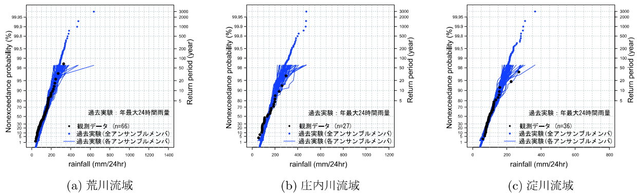
図-8 年最大 24 時間降水量の確率プロットの比較 (黒点: 観測降雨, 青点: d4PDF 過去実験の全アンサンブルメンバ, 青細線: d4PDF 過去実験の 60 年ごとのアンサンブルメンバ)
