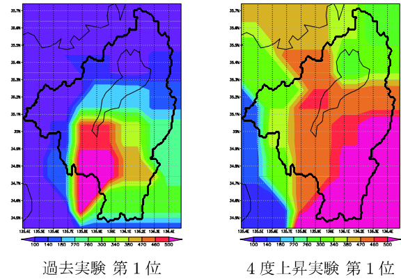
図-14 枚方地点上流域に最大クラス洪水をもたらした d4PDF の 24 時間雨量の空間分布
