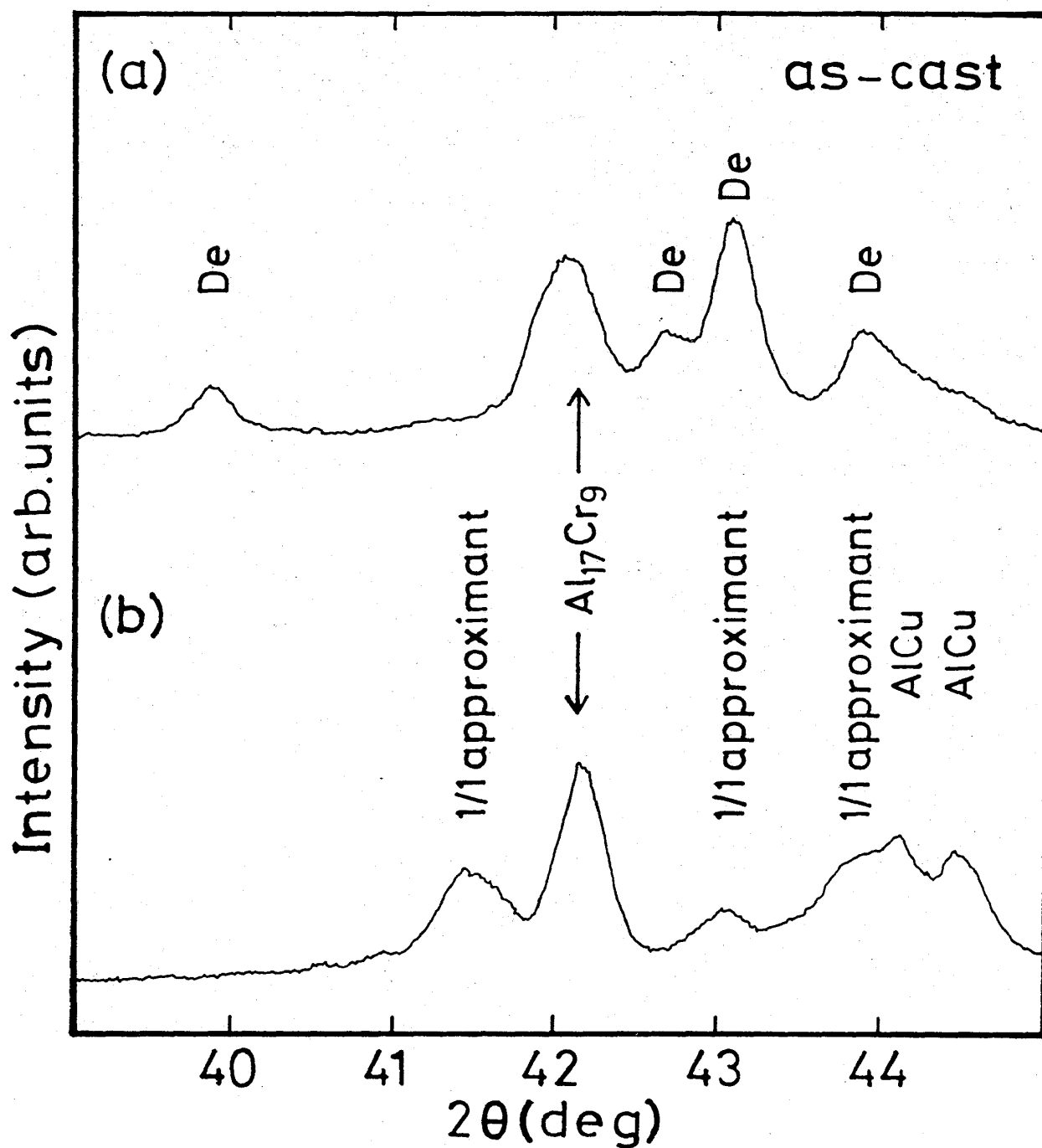
図Ⅱ-5; 2\theta = 39 \sim 45^\circ 付近を走査速度 0.25^\circ/\text{min} で測定した \text{Al}_{70}\text{Cu}_{10}\text{Cr}_{20} 合金 (a) と \text{Al}_{65}\text{Cu}_{20}\text{Cr}_{15} 合金 (b) の as-cast 試料の X 線粉末回折パターン。 \text{Al}_{65}\text{Cu}_{20}\text{Cr}_{15} 合金の as-cast 試料には De 相のピークは認められない。
