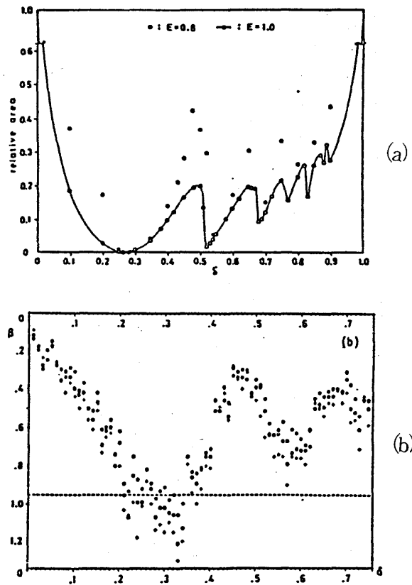
Fig. 1 (a) (q_1, p_1) 断面におけるカオス領域の質量比依存性。実線又はプロットより上の領域が全面積に対するカオス領域の相対面積をあらわす。
