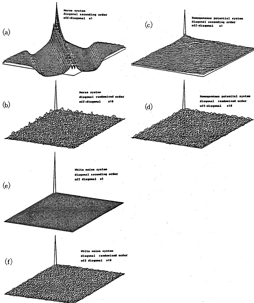
Fig. 3 2次元相関関数
