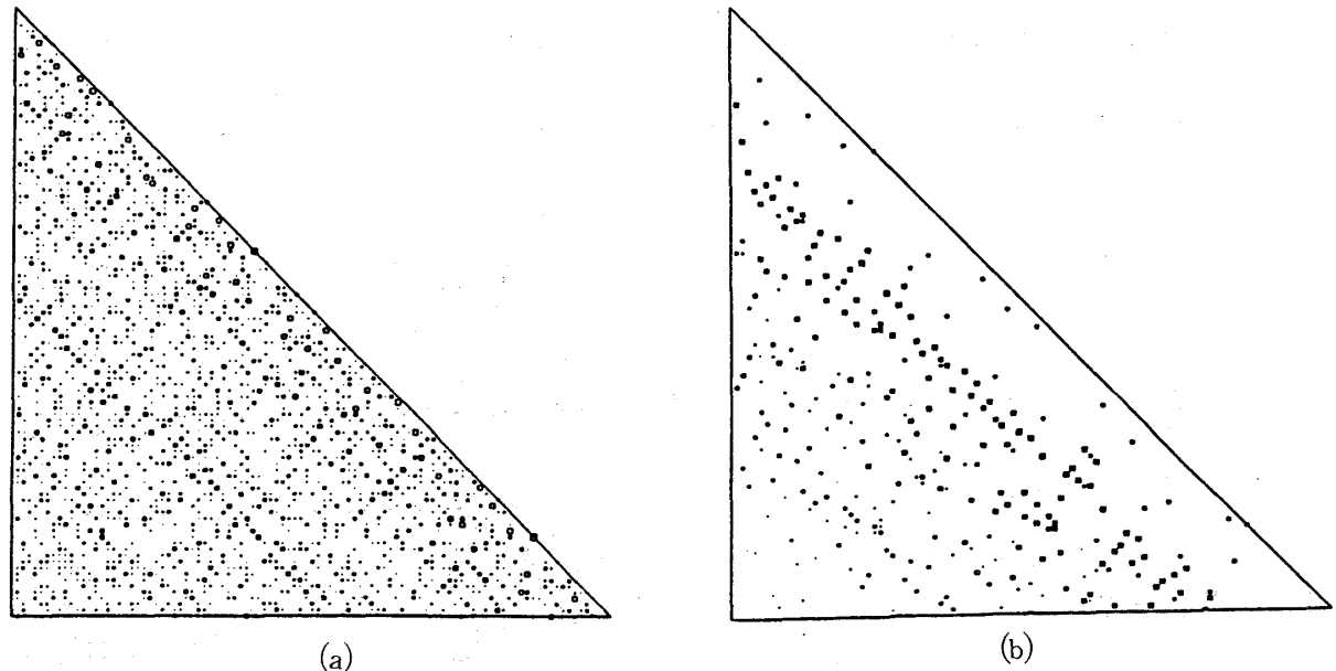
Fig. 2 空間的値分布。四角の大きさは行列要素の値の大きさに比例。黒が正、白が負に対応。(a) モース系 (b) 4次同次系
