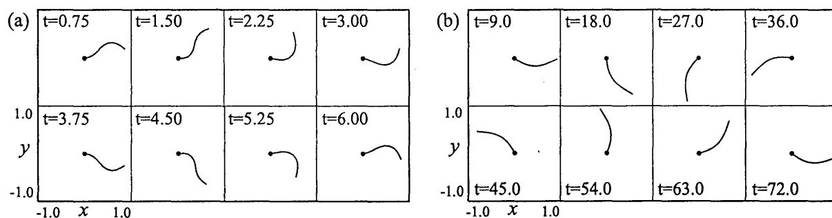
図 1: 臨界を越えたある流量におけるチューブの運動を、各時刻 t におけるスナップショットとして表示した。黒丸は吸い込み口を表す。(a) 吸い込み口の方を固定したチューブは左右に振動し始める。(b) 吸い込み口の方を自由にしたチューブは回転し始める。
