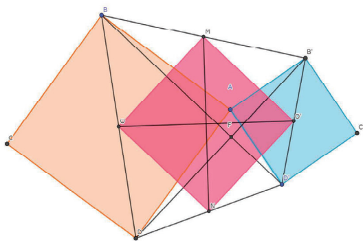
図 7 正方形 ONO'M
