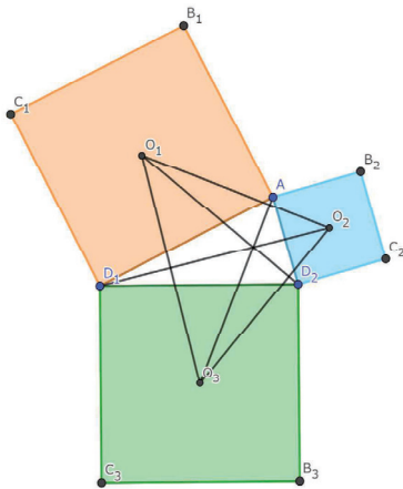
図 11 \triangle O_1O_2O_3
