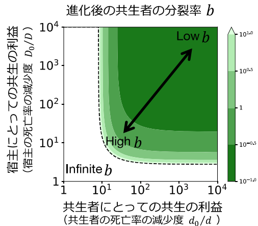
図2：共生者による分裂率の進化
