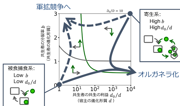
図3：宿主と共生者の共進化動態
