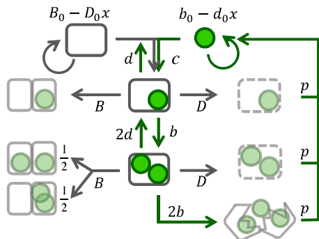
図 1：個体群動態のモデル
