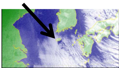
Fig. 3 大気中のカルマン渦①
