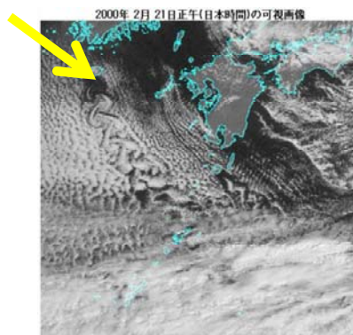
Fig. 4 大気中のカルマン渦②
