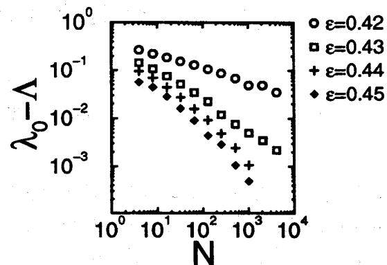
図 10: \lambda_0 と \Lambda の比較
