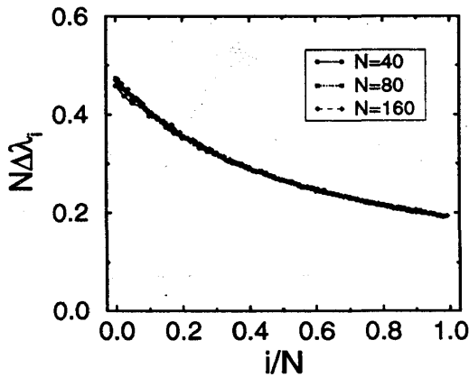
図 5: a = 1.99, \epsilon = 0.25 の時の N\Delta\lambda_i
