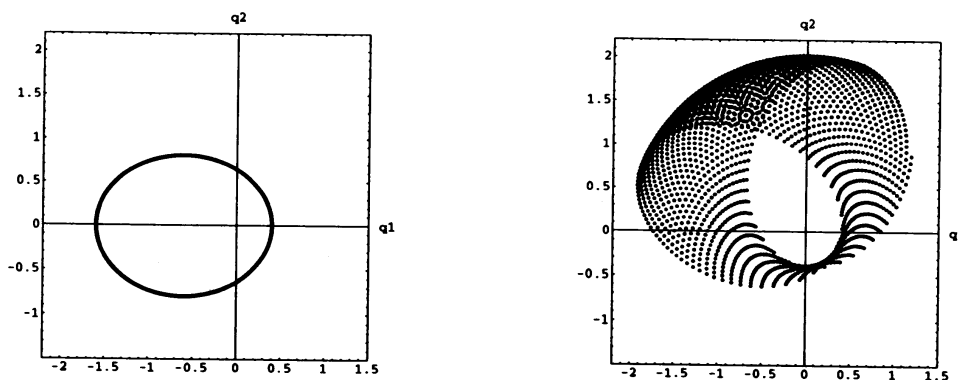
図 3: ケプラー問題の厳密解 (左) と数値解 (右). ( \tau = 0.1 )
