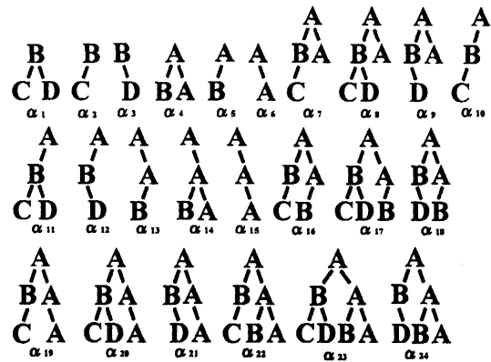
図4: 重複を取り除いた部分木列 SFA(T_A)
