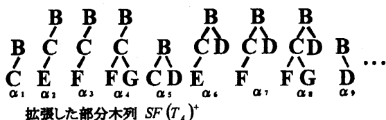
図13:拡張した部分木列 SF(T_A)^+ の例
