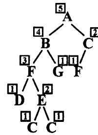
図6: 構文解析木の要素の次数 R(\alpha_n) の例 O(\alpha_n) は次の式で求められる。
