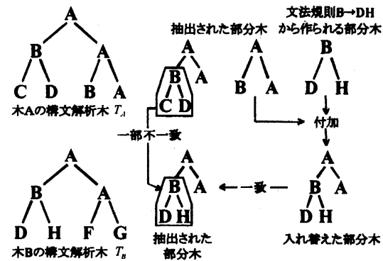
図5: 部分木の拡張の例
