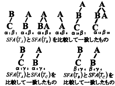
図11: 重複を取り除いた部分木の一致
