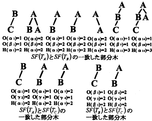
図9: 比較結果の O(\alpha_n) と H(\alpha_n)
