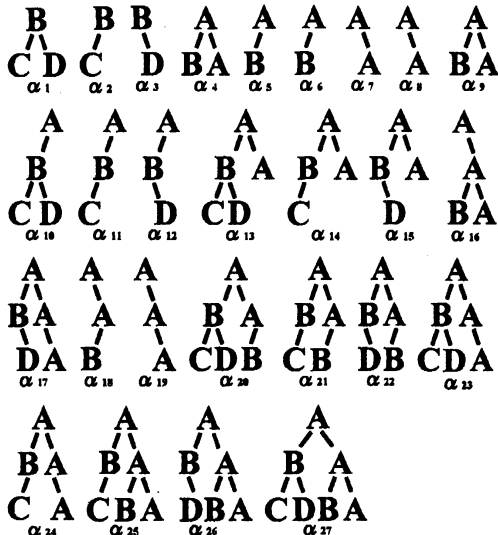
図3: 構文解析木 T_A の部分木列 SF(T_A)
