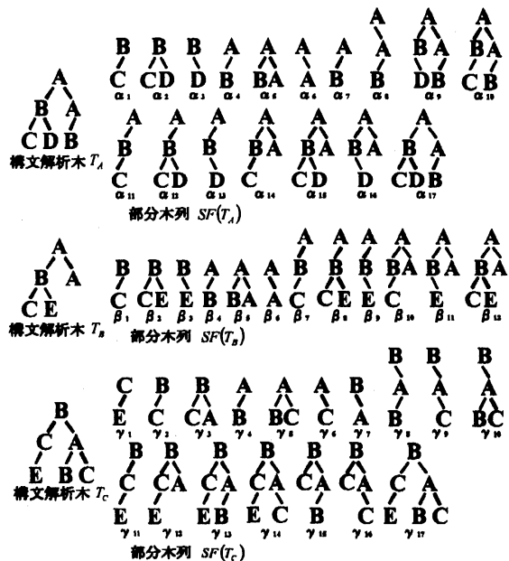
図7: T_A, T_B, T_C の部分木抽出
