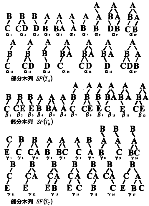
図10: 重複を取り除いた部分木列
