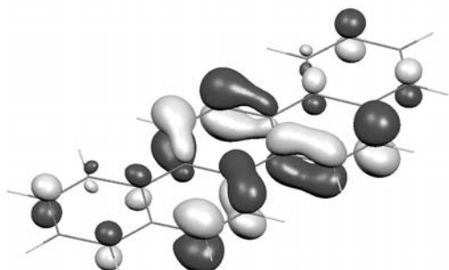
(a) LUMO
