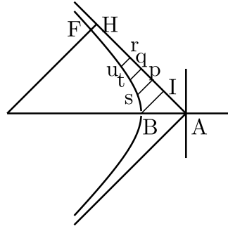
図 1. 直角双曲線と漸近線
