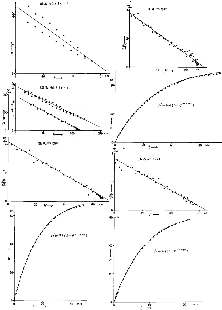
第4圖 水頭と湧出量又は水位上昇速度との關係(正常例)
