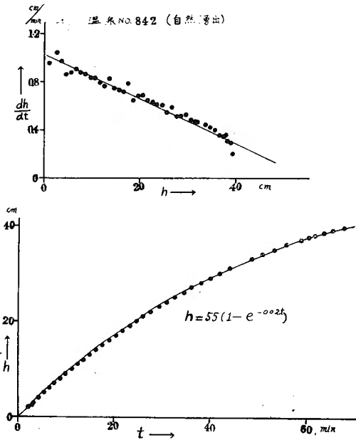
第7図 自然湧出温泉 No. 842 の正常湧出曲線
