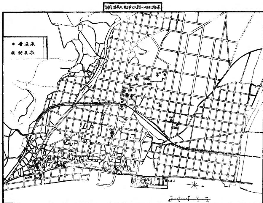
第 1 圖 水 頭 效 果 調 査 泉 の 位 置
