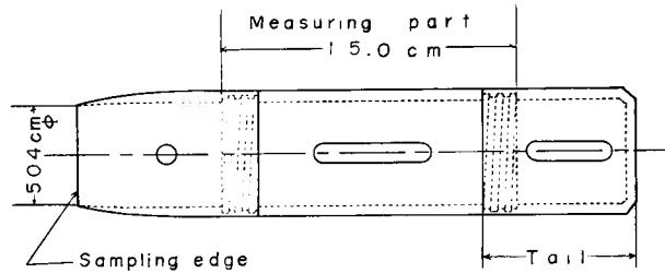
Fig. 1. Snow sampler.
