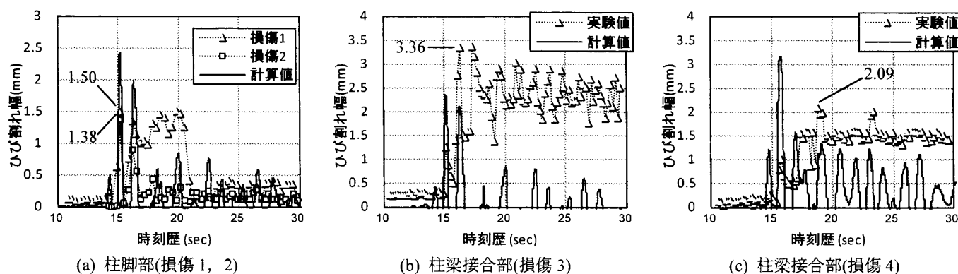
図 4 ひび割れ幅の時刻歴 (JMA-Kobe 波 100%加振)
