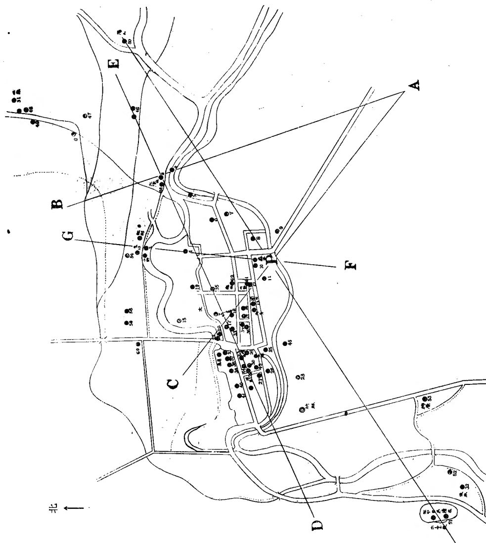
第1圖 内ノ牧温泉分布（数字は町役場温泉臺帳の所載順につけた温泉番號），又氏名は伊木博士報文中の温泉位置，ABは筆者想定のカルデラ裂弱線
