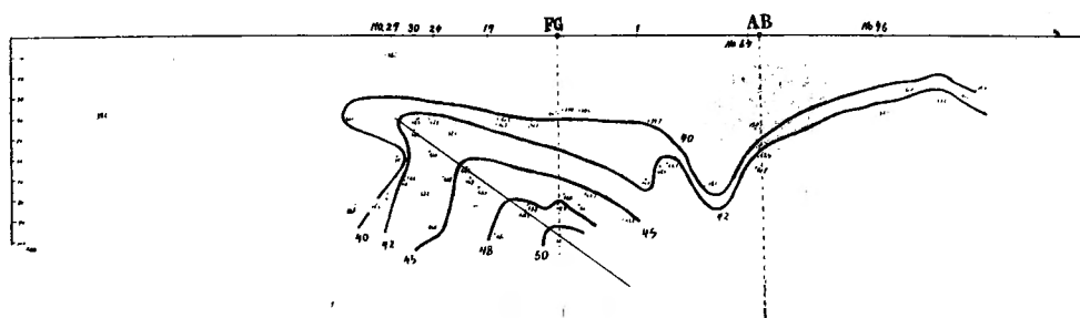
第4圖 垂直斷面上の温度分布
