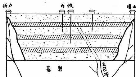
第8圖 内ノ牧温泉地下狀態想像圖
