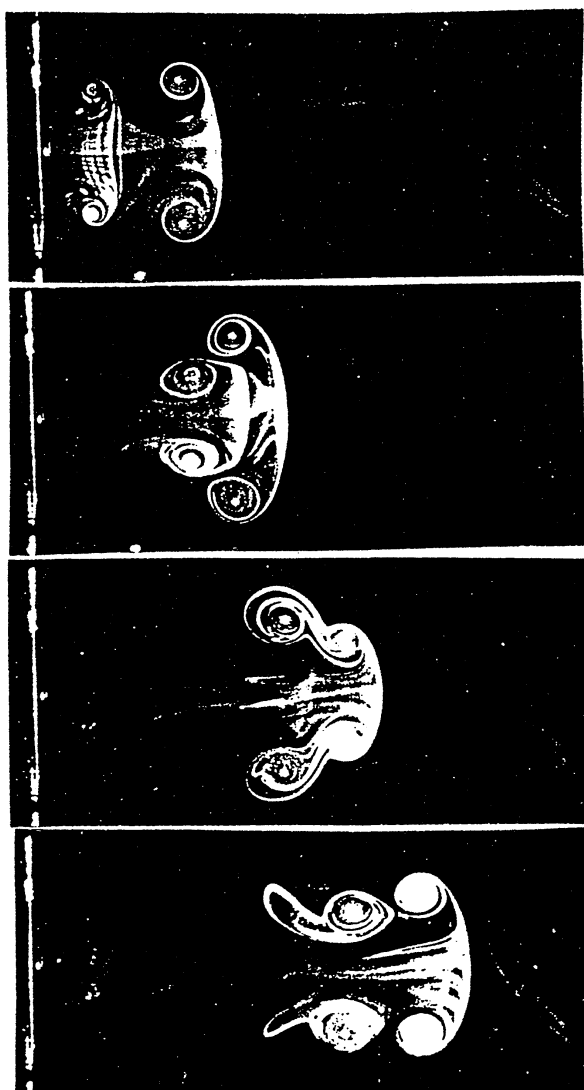
図1. 渦輪の変形
