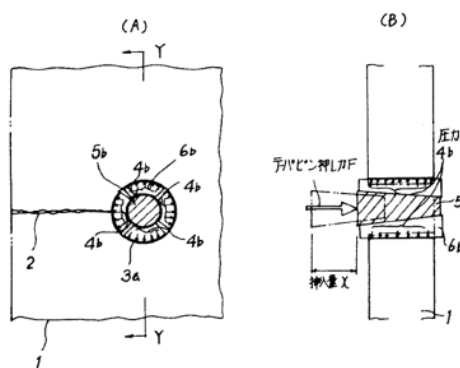
図-7 テーパーピンを用いた 亀裂進展抑止方法 3)
