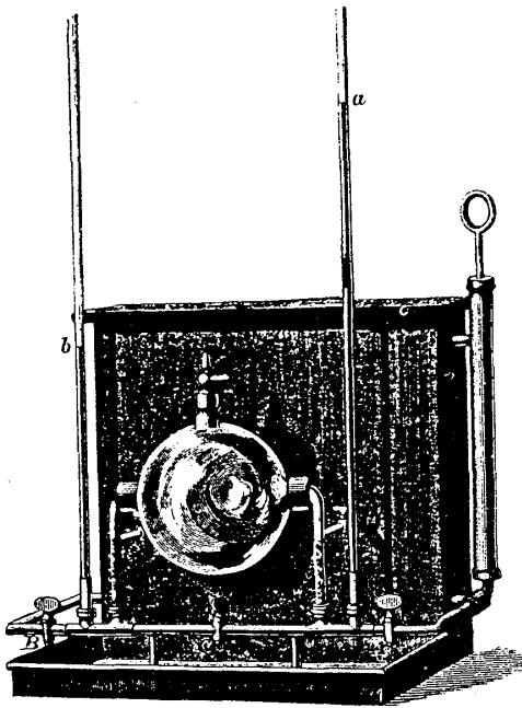
図－8 Lodgeのライデン瓶モデル
