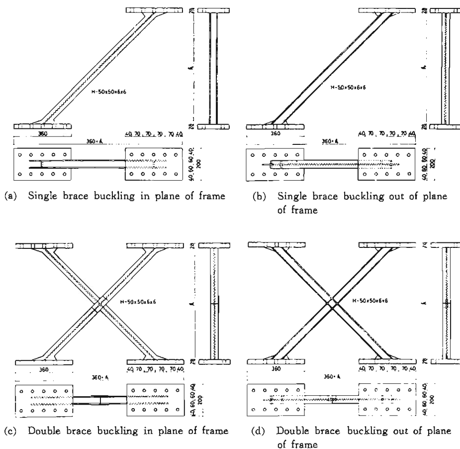
Fig. 3. Specimens
