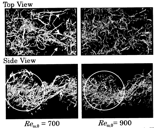
図10 時間発展乱流混合層における第二不変量の等値面 ( Q^* = 0.03 , t = 130 )
