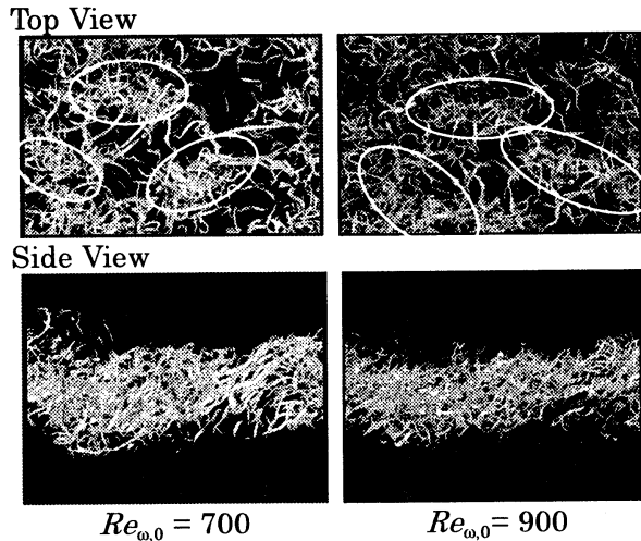
図 9 時間発展乱流混合層における第二不変量の等値面 ( Q^* = 0.03 , t = 90 ).
