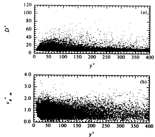
図 14 Channel 乱流におけるコヒーレント微細渦の直径(a)及び最大周方向速度(b) ( Re_{\tau} = 400 ).
