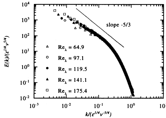
図 2 三次元エネルギー・スペクトル
