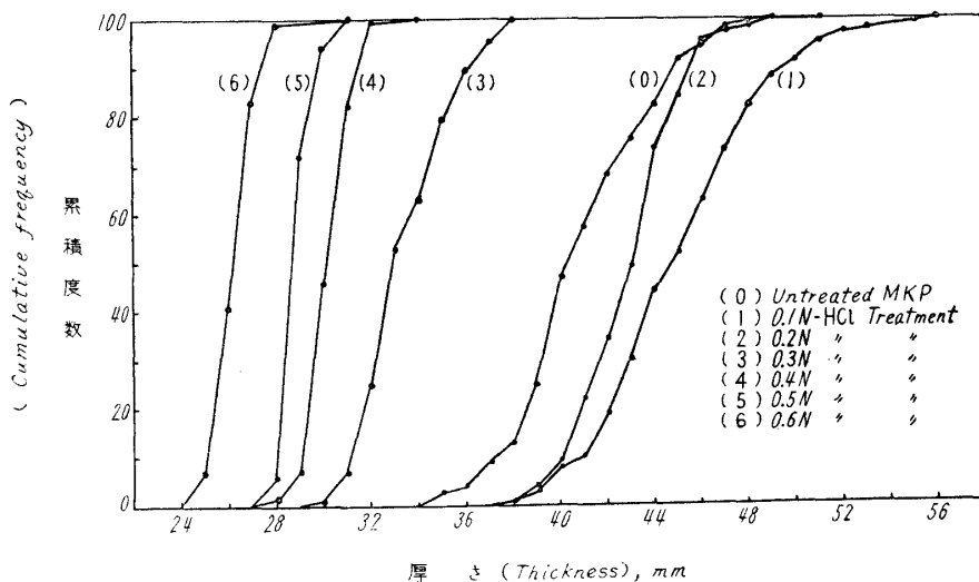
Fig. 1. マーセル化KPの加水分解がシートの厚さの度数分布に及ぼす影響
