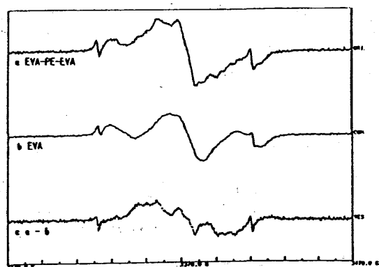
■1 400kGy \gamma -線(空气中)照射直後のEVA-PE-EVAとEVAのESRスペクトル
