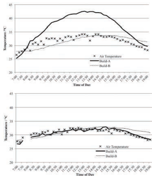
図-9 ペンキに微小セラミック球を混ぜる前(上図)と混ぜた後(下図)の金属製屋根の温度変化(Ohkawa, et al., 2011)。×印は気温、細線は既に微小セラミック球入り塗料を塗布した屋根の表面温度変化、太線は塗料塗布前後の温度変化。微小セラミック球入りの塗料塗布により、日射の熱エネルギー吸収効果に変化が現れ、実に10度程度の表面温度の違いが生まれたことがわかる。
