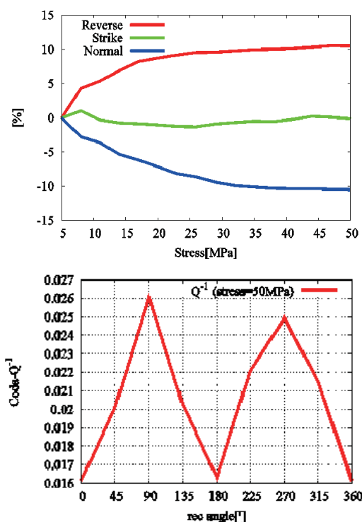
図-8 応力変化とQ値の変化(百分率)の関係(上図)。図7に対応した、逆断層(赤線)、正断層(青線)、横ずれ断層(緑)を想定している。Q値変化を推定する方向と応力の最も大きくなる方向の関係(下図)。上図からは、方位で平均した応力値に従うQ値の変化が期待されることがわかる。下図からは、Q値の変化が、働く応力の方位に依存することも示している。
