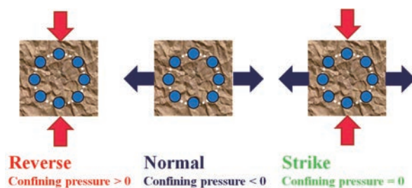
図-7 2次元の正方形地殻モデルに与えた、逆断層（左）、正断層（中央）、横ずれ断層（右）を引き起こす応力変化（岡本、2011）。図中の青丸はシミュレーション結果となる地震波形を求める位置を示す。入力となる地震波には平面波を仮定し、一方向からの入射に対するQ値を推定する。全方位からの入射に対するQ値を平均して、Q値が応力により変化する（Q値の応力依存性と呼びます）を確認した。
