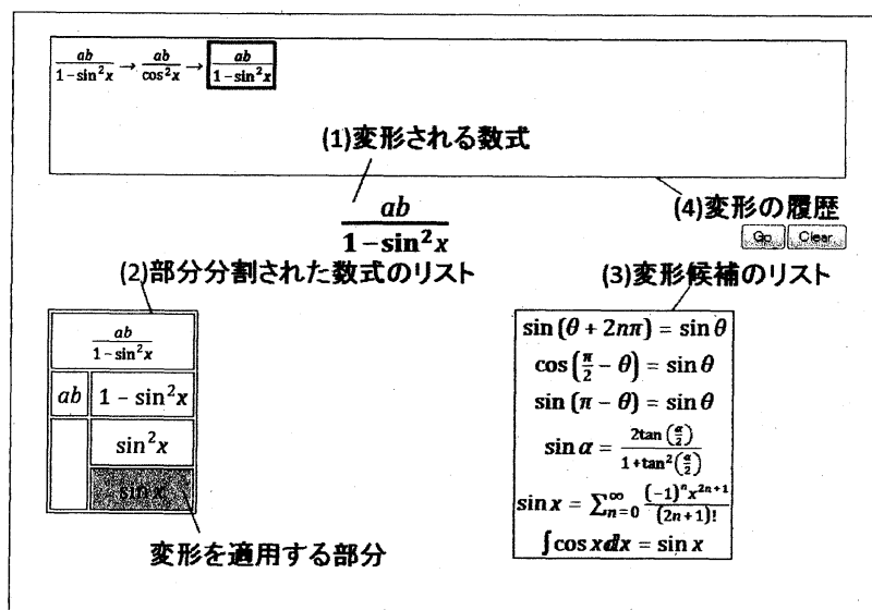
図 3: インタフェース
