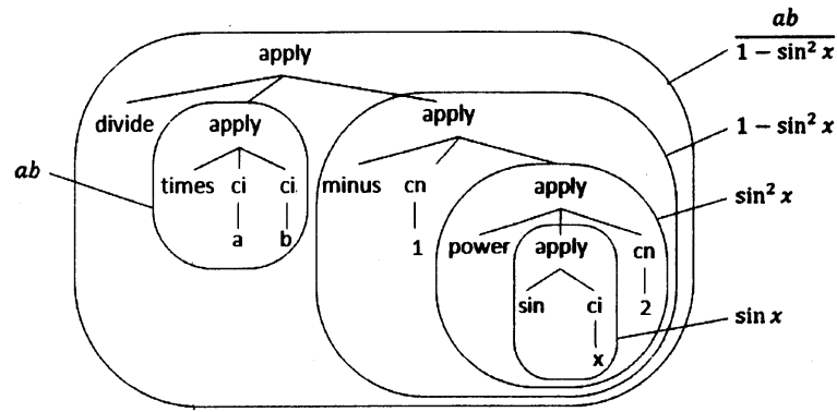
図 2: \frac{ab}{1 - \sin^2 x} の木
