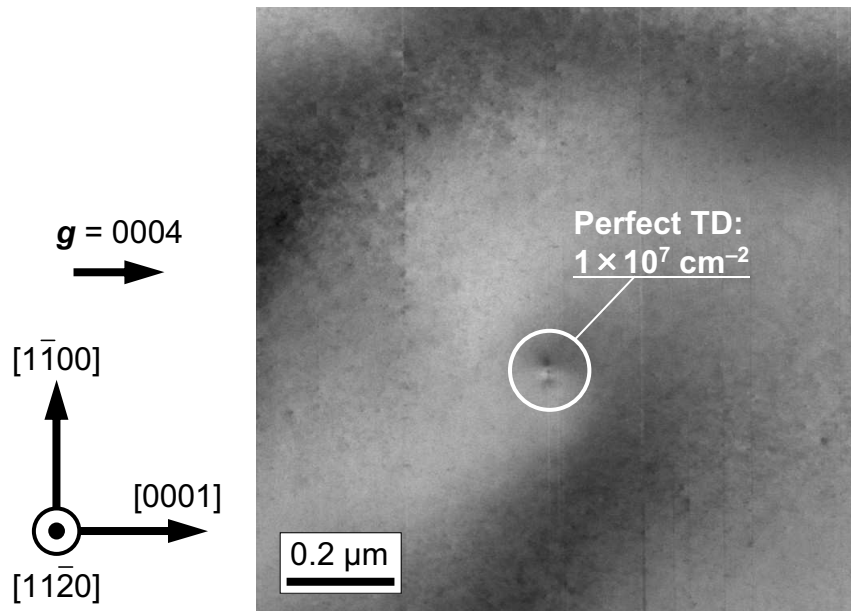
(b) \mathbf{g} = 0004
